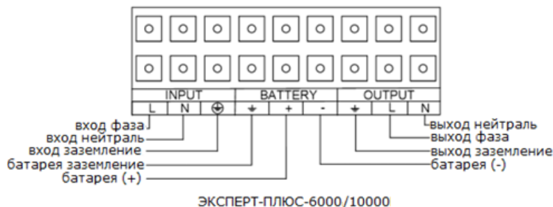
Рис. 4-2 – Входная и выходная схема подключения клеммного блока
